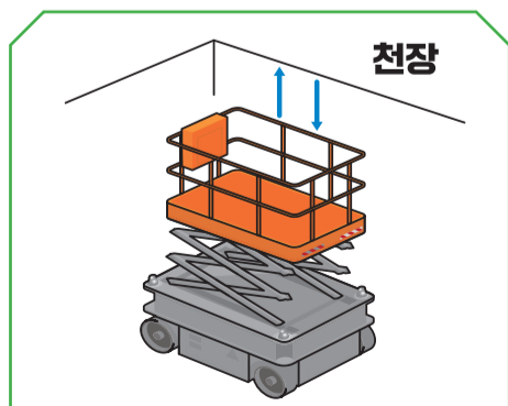
고소작업대 스마트 안전장치 (비접촉 과상승방지장치)
